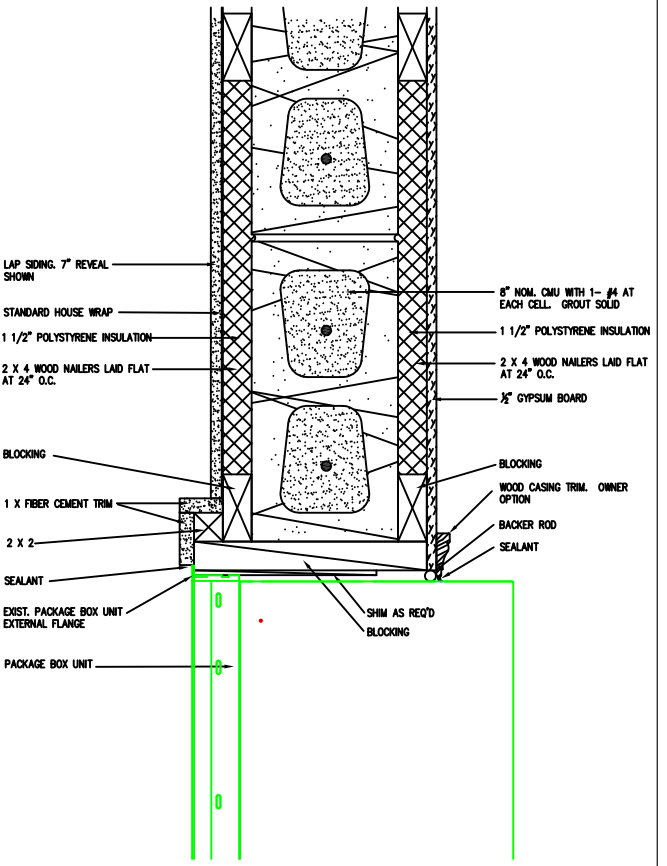
JAMB DETAIL
